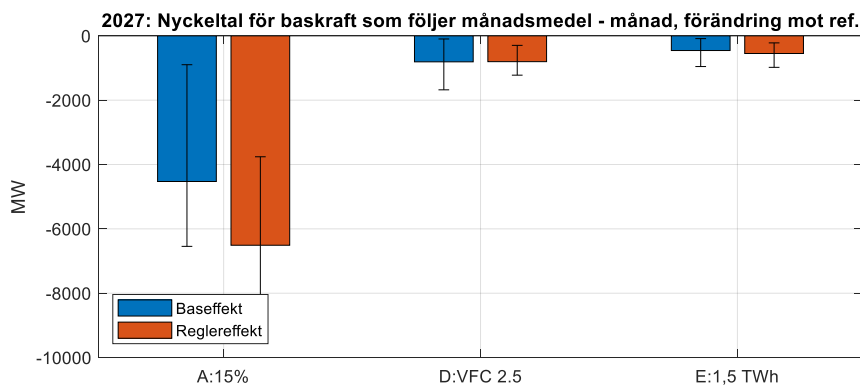
Figur 21. Förändring av baseffekt och reglereffekt över månadshorisonten vid olika miljöalternativ jämfört med referensalternativet år 2027. De svarta klammarna visar spridningen över väderåren. Källa: Svenska kraftnät.
