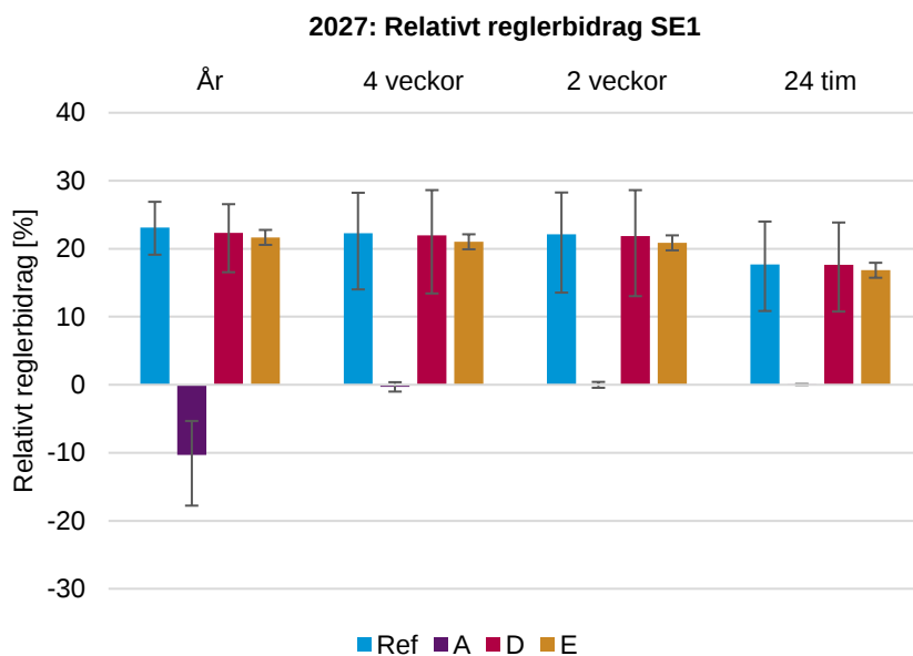
Figur 32. Relativa reglerbidraget från vattenkraft i elområde SE1 år 2027 med olika miljöalternativ. Medelvärde över alla väderår och de svarta klamrarna visar spridningen mellan väderår. Källa: Svenska kraftnät.
