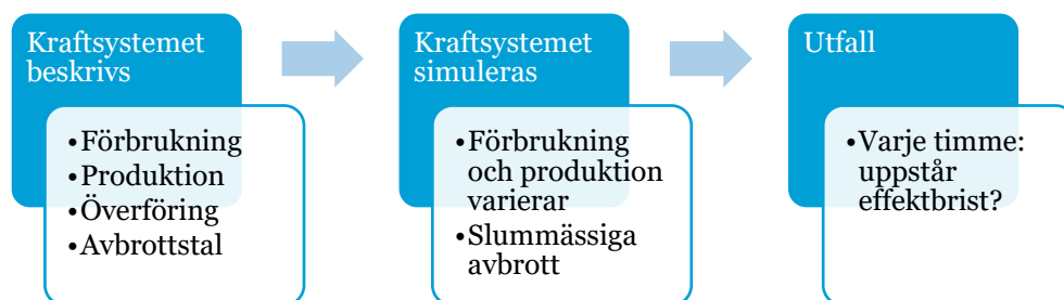
Figur 44. Schematisk beskrivning av den probabilistiska metoden. Källa: Svenska kraftnät.
