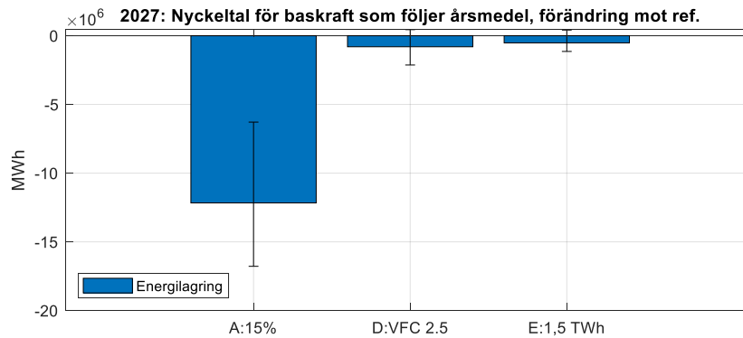
Figur 39. Förändring mot referens av energilagring över årshorisonten år 2027. Spridningen över väderåren visas med de svarta klamrarna. Källa: Svenska kraftnät.
