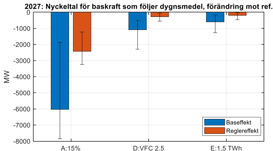
Figur 36. Förändring av bas- och reglereffekt över dygnshorisonten år 2027 för olika miljöalternativ i jämförelse med referensalternativet. Spridningen över väderåren visas med de svarta klamrarna. Källa: Svenska kraftnät.
