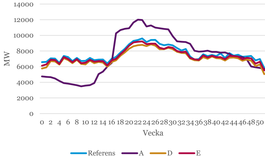
Figur 47. Vattenkraftens medeleffekt per vecka för 2045 Elektrifiering förnybart. Källa: Svenska kraftnät
