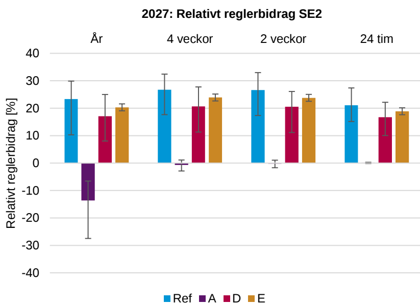
Figur 33. Relativa reglerbidraget från vattenkraft i elområde SE2 år 2027 med olika miljöalternativ. Medelvärde över alla väderår och de svarta klamrarna visar spridningen mellan väderår. Källa: Svenska kraftnät.
