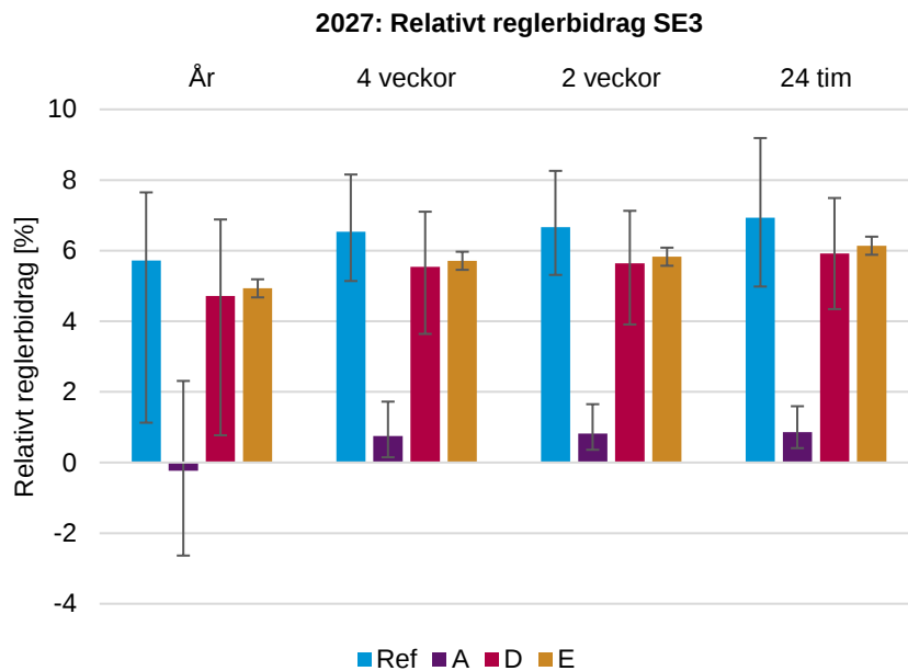
Figur 34. Relativa reglerbidraget från vattenkraft i elområde SE3 år 2027 med olika miljöalternativ. Medelvärde över alla väderår och de svarta klamrarna visar spridningen mellan väderår. Källa: Svenska kraftnät.
