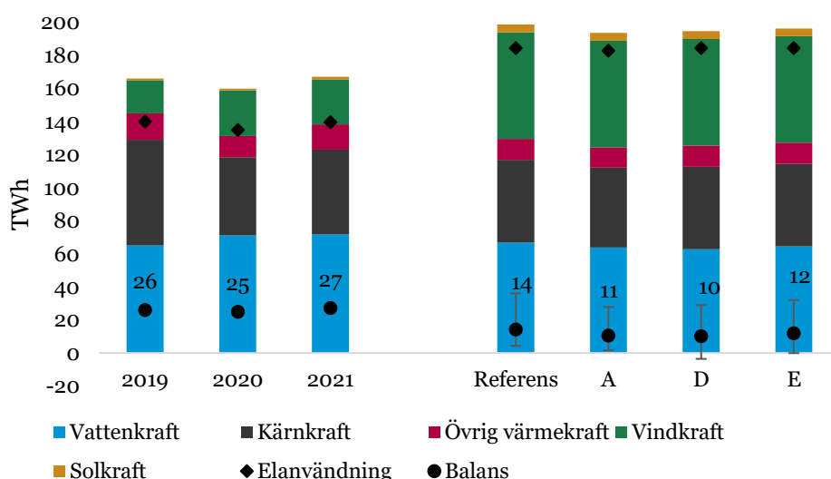
Figur 7. Produktion, elanvändning och resulterande energibalans (TWh) i Sverige per miljöalternativ A, D och E för år 2027. De svarta klammarna visar inom vilket spann årsenergibalansen ligger med hänsyn till de 26 väderår som använts. Källa för historiska år: Energiföretagen och övrig data Svenska kraftnät.
