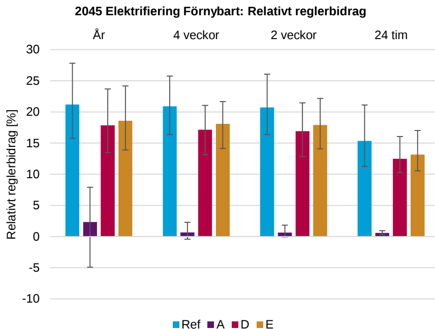
Figur 16. Relativa reglerbidraget från svensk vattenkraft för Elektrifiering Förnybart 2045 med referens- och miljöalternativ A, D och E. Medelvärde över alla väderår och de svarta klammarna visar spridningen mellan väderår. Källa: Svenska kraftnät.
