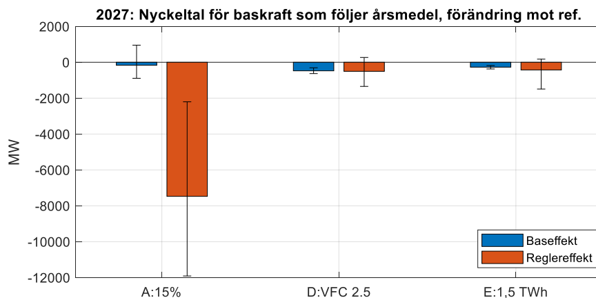
Figur 38. Förändring mot referens av baseeffekt och reglereffekt över årsshorisonten år 2027. Spridningen över väderåren visas med de svarta klamrarna. Källa: Svenska kraftnät.
