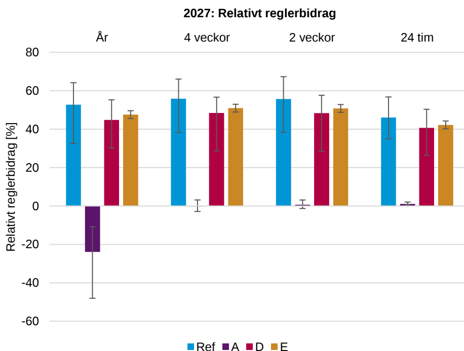
Figur 14. Relativa reglerbidraget från svensk vattenkraft år 2027 med referens- och miljöalternativ A, D och E. Medelvärde över alla väderår. De svarta klamrarna visar spridningen mellan väderår. Källa: Svenska kraftnät.
