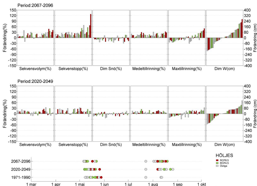
Figur 3.16. Procentuell förändring för Höljesdammen av sekvensvolym, sekvenstopp, dimensionerande snömagasin, medeltillrinning, maximal tillrinning vid dimensioneringstillfället, samt förändring av dimensionerande vattenstånd i cm enligt 36 st olika klimatsimuleringar gällande perioden 2067-2096 (över) och 2020-2049 (under). Referensperioden som beräkningarna jämförs mot är 1971-1990. Längst ner visas tidpunkt för dimensionerande vattenstånd för de tre beräkningsperioderna.
