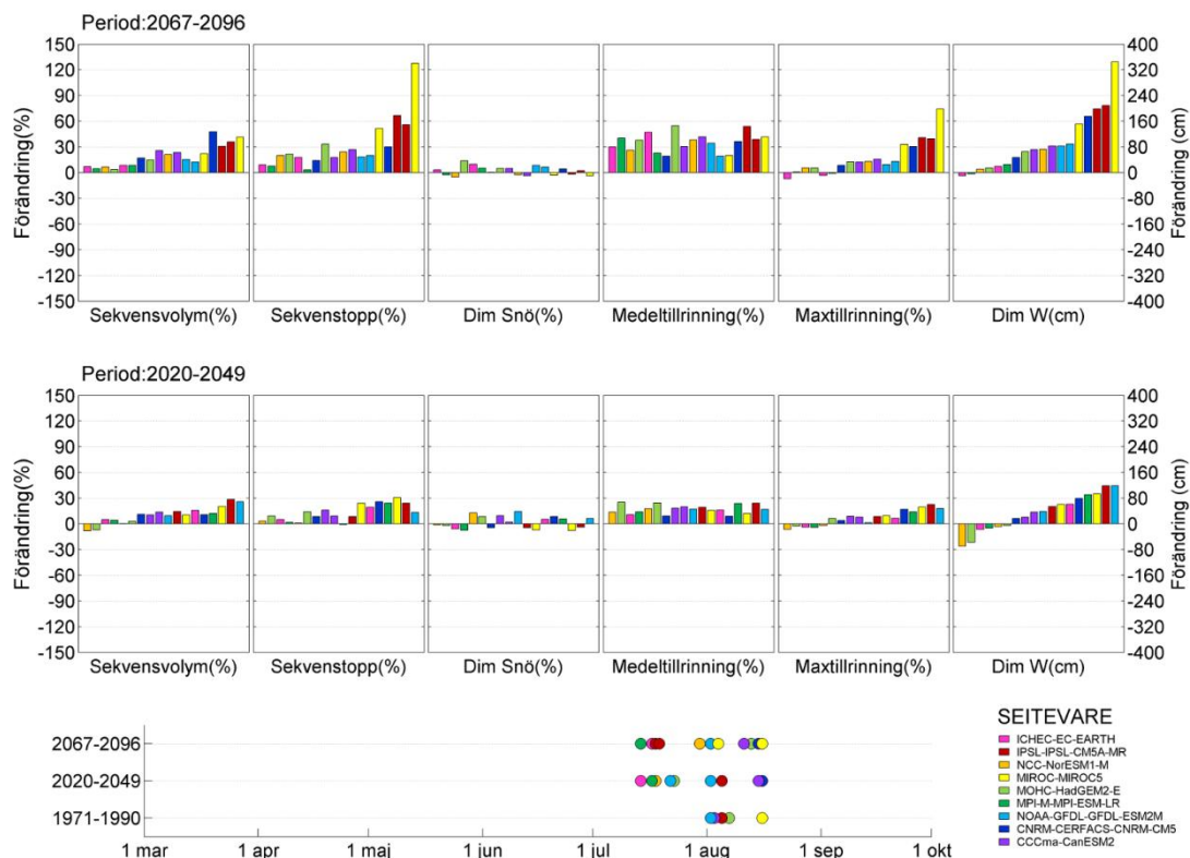
Figur 6.3. Procentuell förändring för Seitevare av sekvensvolym, sekvenstopp, dimensionerande snömagasin, medeltillrinning, maximal tillrinning vid dimensioneringstillfället, samt förändring av dimensionerande vattenstånd i cm gällande perioden 2067-2096 (över) och 2020-2049 (under). Referensperioden som beräkningarna jämförs mot är 1971-1990. Längst ner visas tidpunkt för dimensionerande vattenstånd för de tre beräkningsperioderna. Samtliga simuleringar är av typ RCP4.5 eller RCP8.5.
