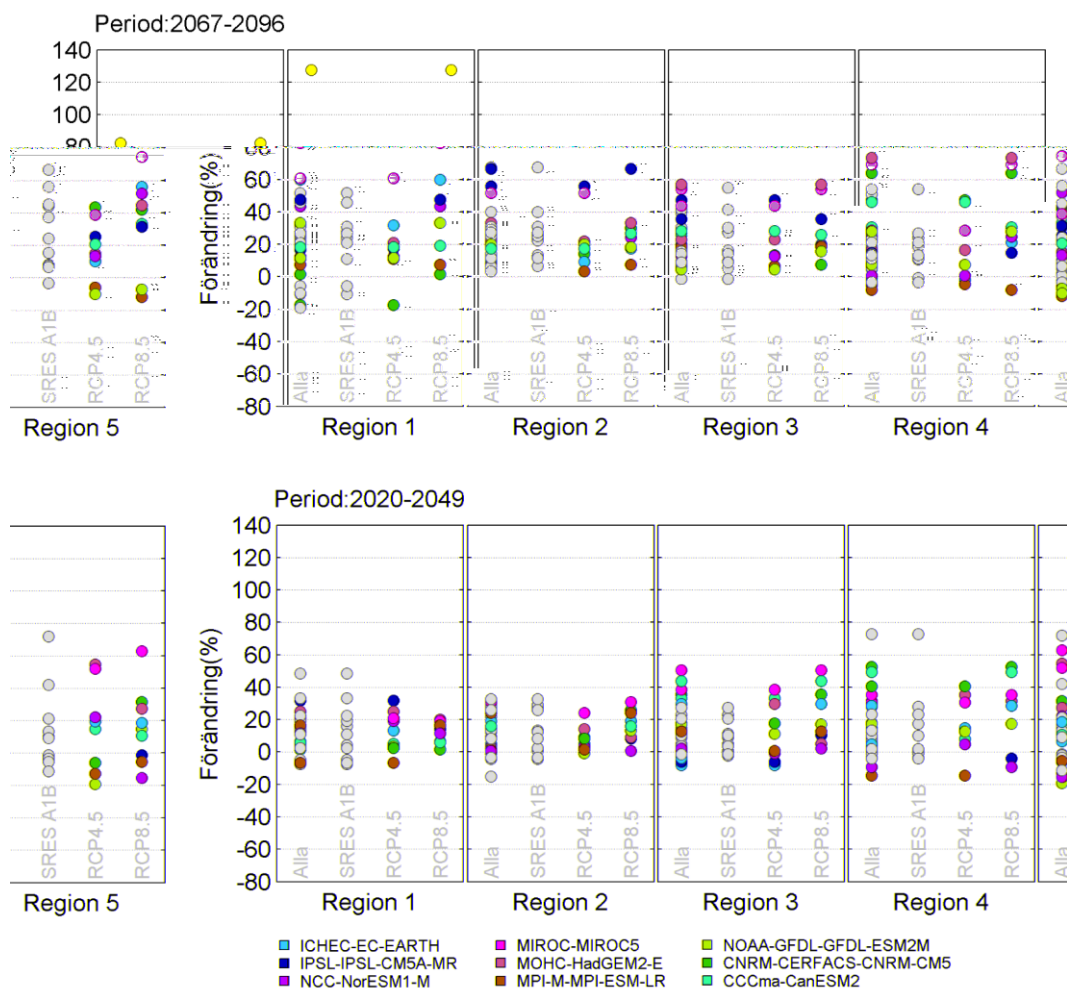
Figur 6.1. Förändring av den dimensionerande nederbördssekvensens maxvärde för perioderna 2067-2096 (övre) och 2020-2049 (undre) jämfört med referensperioden 1961-1990. Resultat baserade på RCP-scenarier redovisas i färg (efter global modell) medan resultat baserade på SRES-scenarier visas i grått.
