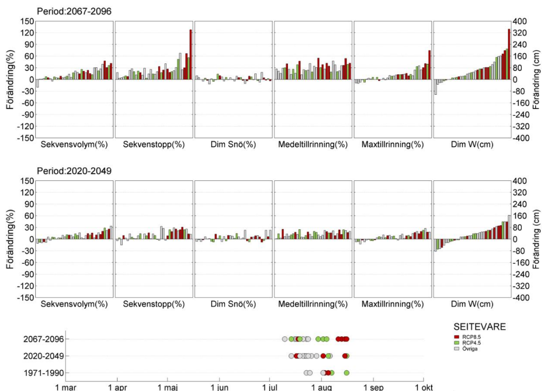
Figur 3.8. Procentuell förändring för Seitevare av sekvensvolym, sekvenstopp, dimensionerande snömagasin, medeltillrinning, maximal tillrinning vid dimensioneringstillfället, samt förändring av dimensionerande vattenstånd i cm enligt 36 st olika klimatsimuleringar gällande perioden 2067-2096 (över) och 2020-2049 (under). Referensperioden som beräkningarna jämförs mot är 1971-1990. Längst ner visas tidpunkt för dimensionerande vattenstånd för de tre beräkningsperioderna.
