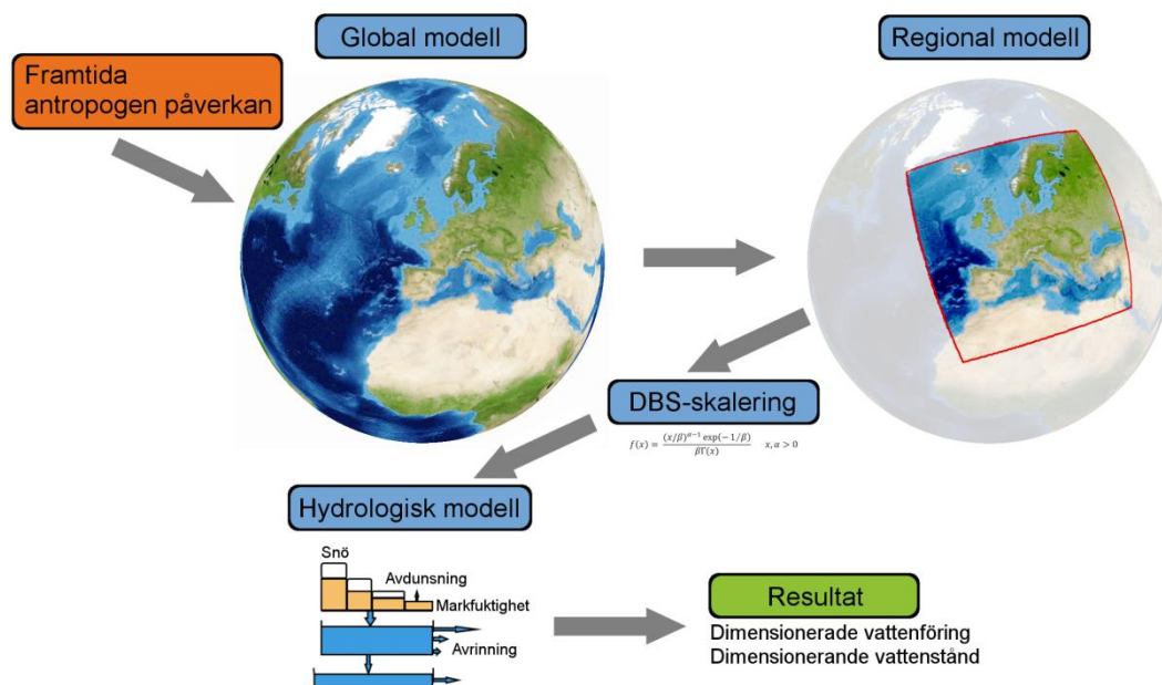
Figur 2.5. Illustration av kopplingen mellan global- och regional klimatmodell samt hydrologisk modell vid studier av klimateffekter på beräkningar för dammanläggningar i flödesdimensioneringsklass I.
